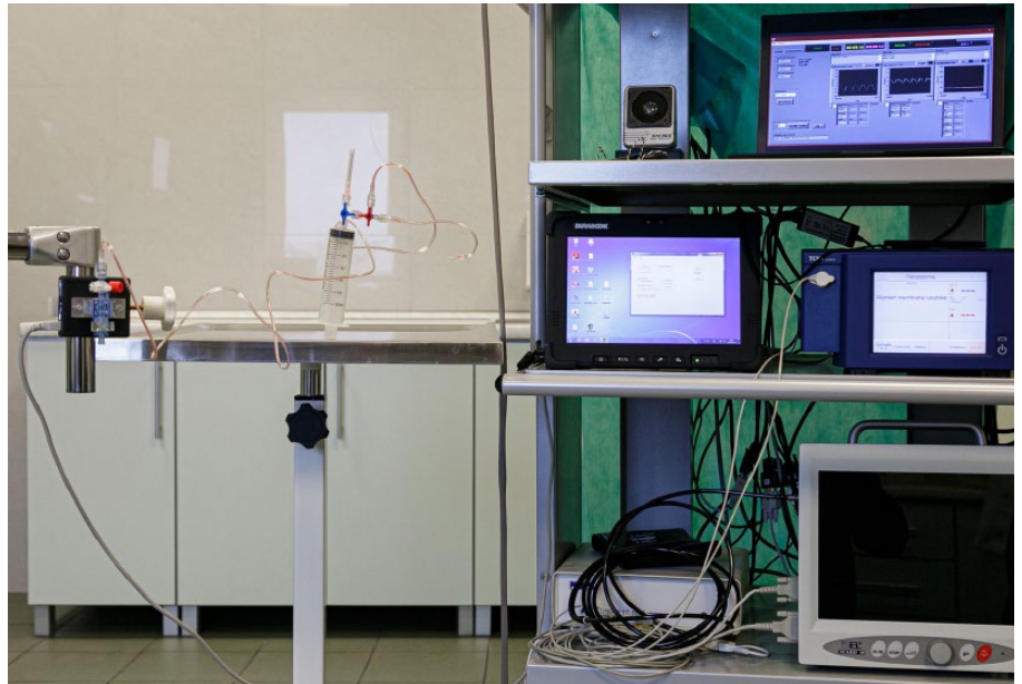
Elektroniczny manometr wykorzystywany do mierzenia ciśnienia opłucnowego
